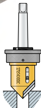
Autosvasatori per interni
